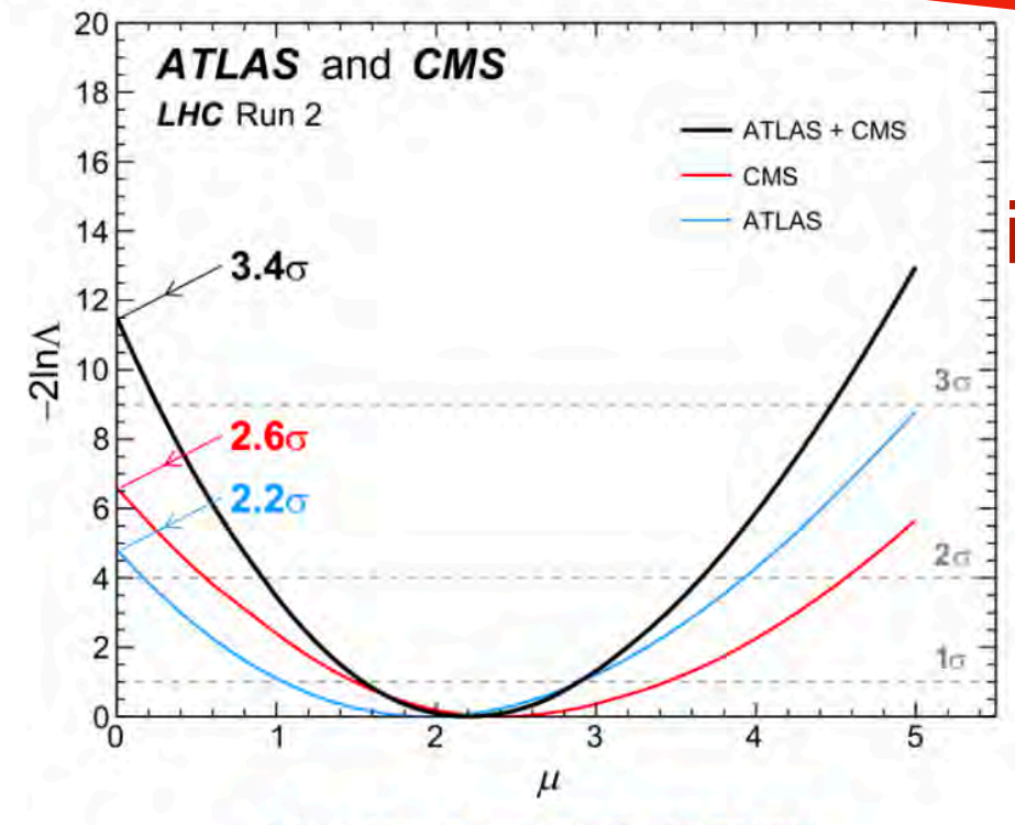
PhysRevLett.132.021803
