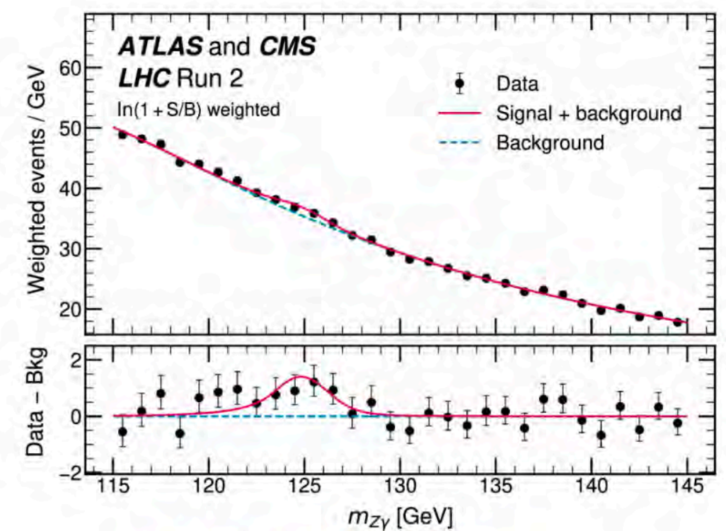
PhysRevLett.132.021803
