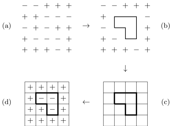
図 1: イジング模型の双対性
